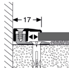
Kübler PPS Champion Star Abschlussprofil Art.-Nr.: 55202xxxx Edelstahloptik 100 cm / 270 cm / 300 cm
