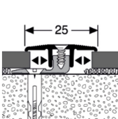
Kübler PPS Champion Star Übergangsprofil Art.-Nr.: 55202xxxx Edelstahloptik 100 cm / 270 cm / 300 cm
