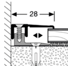
Kübler PPS Champion flex Abschlussprofil Art.-Nr.: 55200xxxx Edelstahl 100 cm / 270 cm / 300 cm
