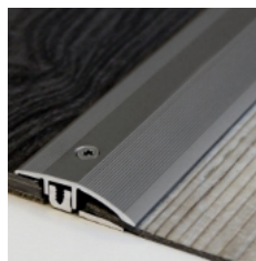
Kübler PPS Champion Star Anpassungsprofil Art.-Nr.: 55202xxxx Edelstahloptik 100 cm / 270 cm / 300 cm
